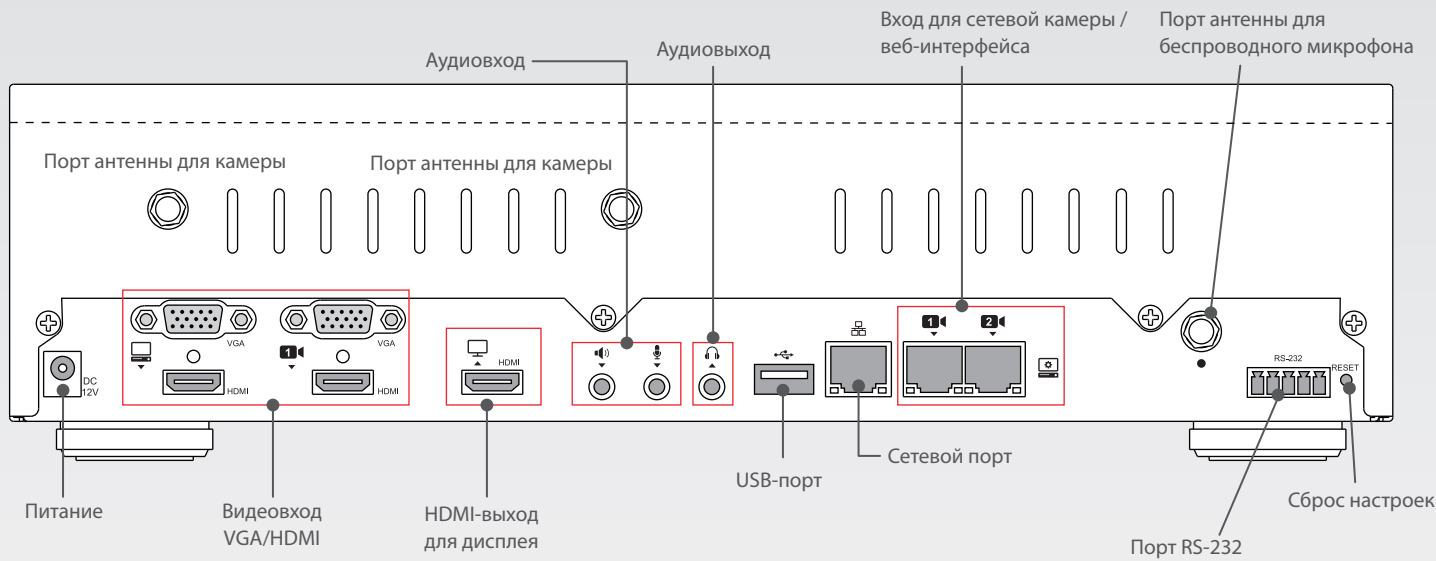
Вид сзади
